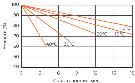
График саморазряда
