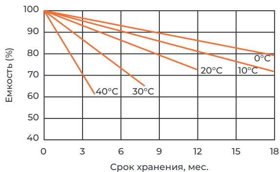
График саморазряда
